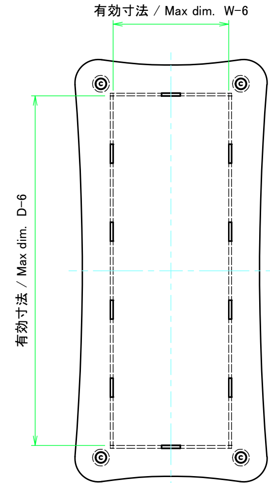
下カバー / Bottom cover
